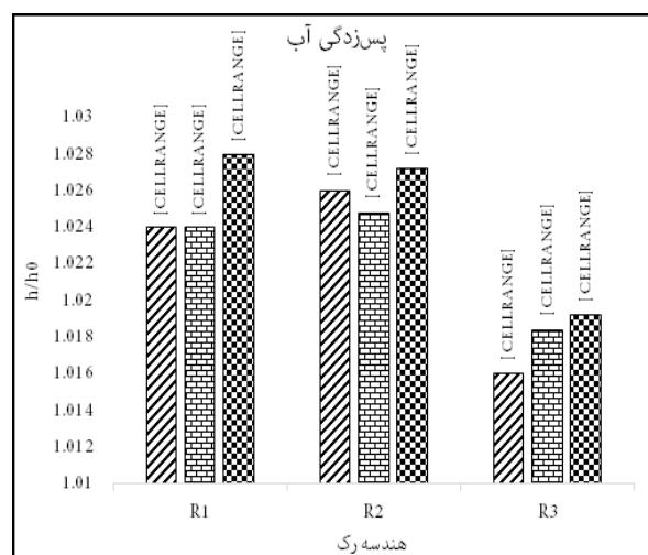
شکل ۹- بررسی تأثیر همزمان منحرف‌کننده‌ها و هندسه آشغال‌گیر در پس‌زدگی آب در جریان بحرانی؛ O1، O2 و O3 به ترتیب سایزهای کوچک، متوسط و بزرگ نیم‌گوی‌ها می‌باشند.
